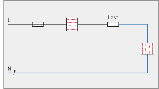
Bild 1: Serieller Fehlerlichtbogen
