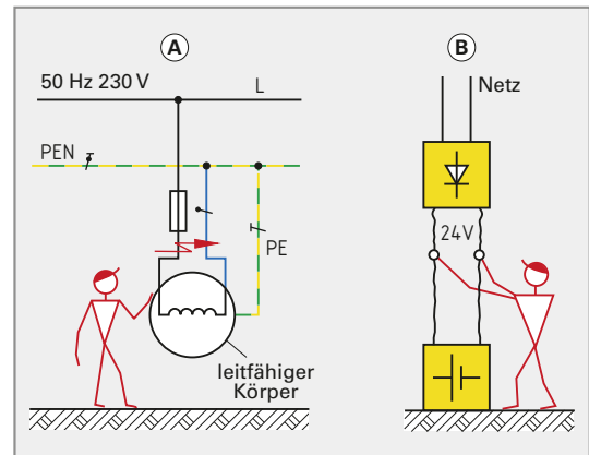
Bild 1: Direktes, indirektes Berühren
