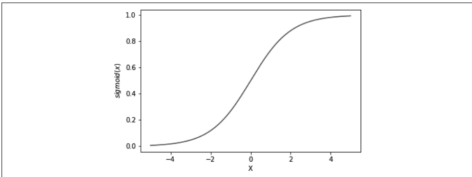
Abbildung 2-9: Grafische Darstellung der sigmoid-Funktion im Bereich zwischen x = -5 und x = 5
