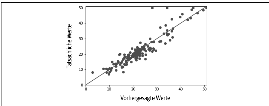
Abbildung 2-6: Vorhergesagte und tatsächliche Werte für unser selbst entwickeltes lineares Regressionsmodell
