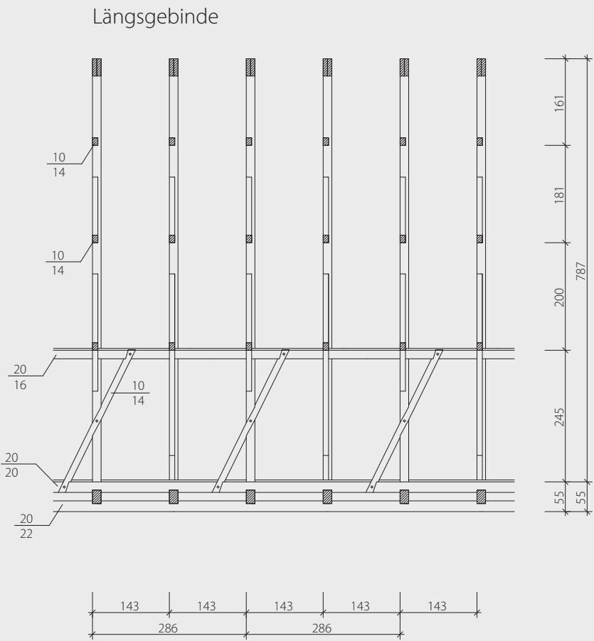
2 Langhausdachwerk, Stuhlwand mit Längsverstrebung.
