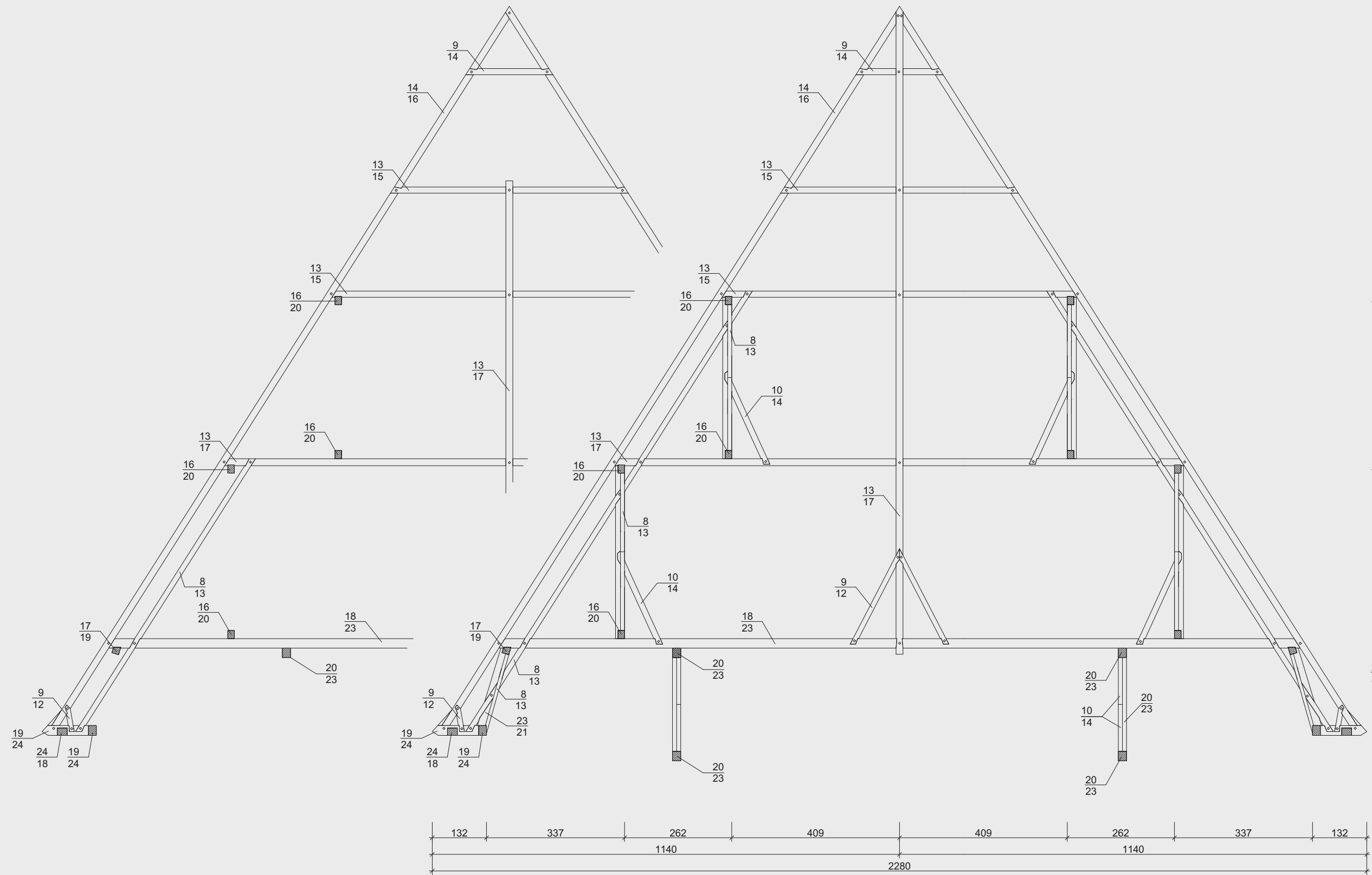
Quergebinde
