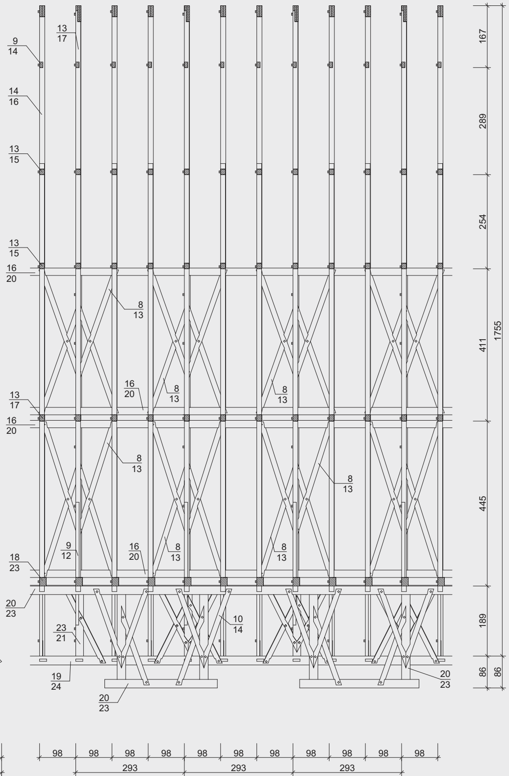
Längsgebinde
