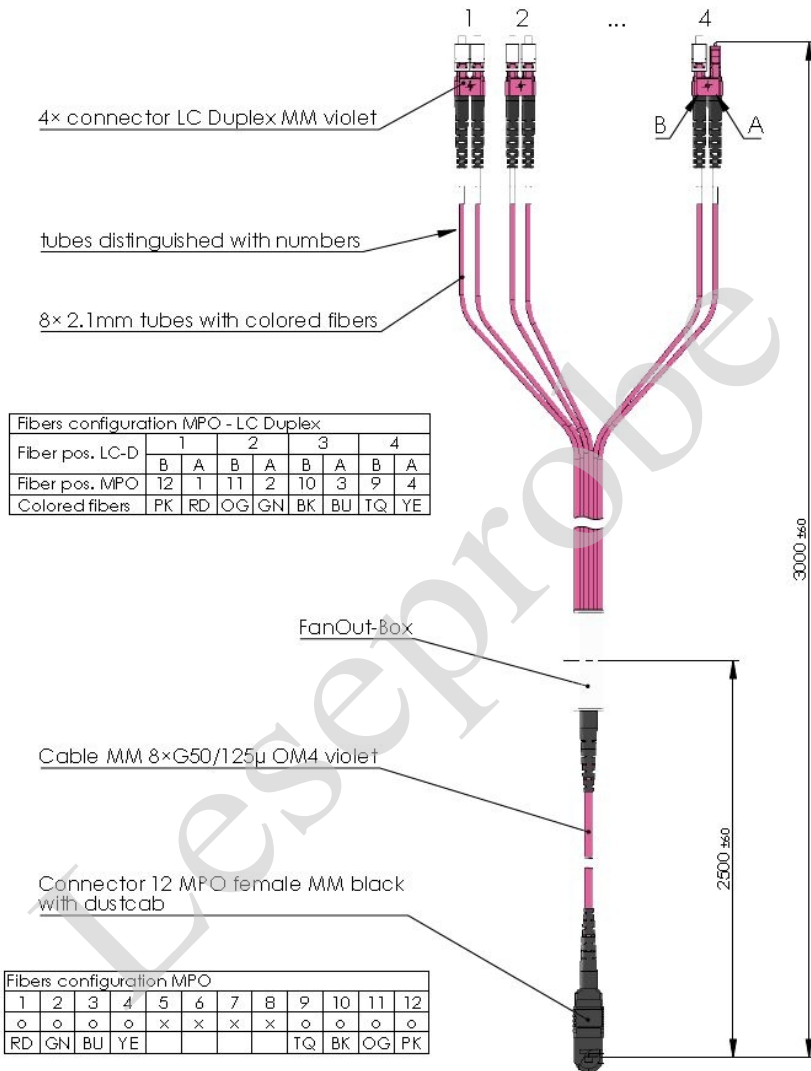
Bild 7.14: Beispiel für ein MPO-Harnesskabel mit nur acht Fasern. Manche Switchanschlüsse für 40 Gigabit Ethernet mit MPO lassen sich auf vier getrennte 10 Gigabit Ethernet-Kanäle aufteilen. Hierfür werden nur acht Fasern benötigt. (Zeichnung: Telegärtner).
