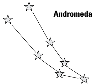
Abbildung 1.2: Der Name Andromeda stammt von einer alten griechischen Prinzessin, die an einen Felsen geschmiedet wurde; daher die Bezeichnung »Frau in Ketten«.
