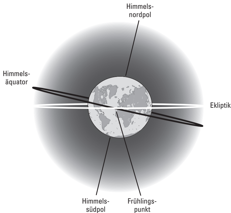
Abbildung 1.3: Die Entschlüsselung der Himmelskugel zur Richtungsbestimmung im All
