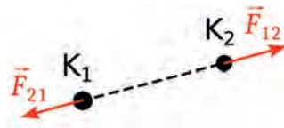
abstoßende Kräfte
