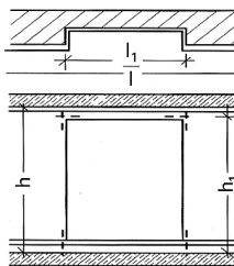
Bild 1.11 j Wenn Vorlage t \times b bzw. Öffnung < 2,5 \text{ m}^2 dann übermessen, bei > 2,5 \text{ m}^2 abziehen.
