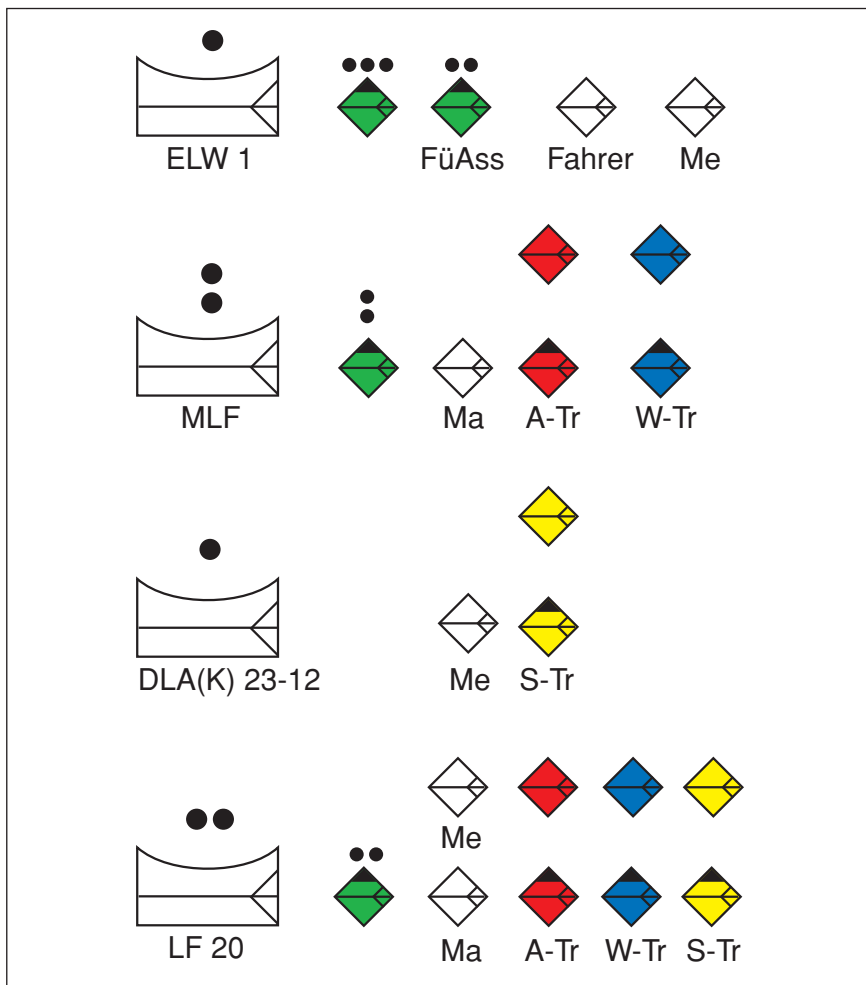
Abbildung 8: Ein Zug mit einem Einsatzleitfahrzeug ELW 1, einem Mittleren Löschfahrzeug MLF, einer Drehleiter DLA (K) 23-12 und einem Löschgruppenfahrzeug LF 20 für die Menschenrettung und Brandbekämpfung im getrennten Einsatz
