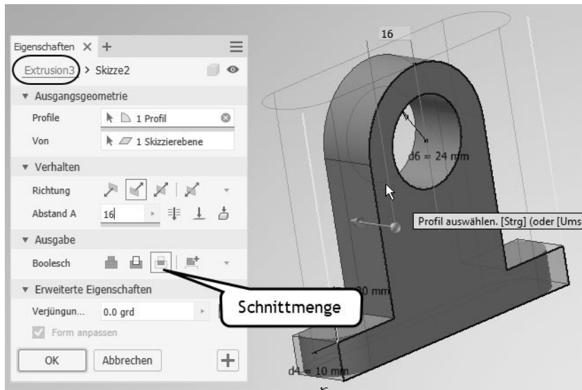
Abb. 1.36: Extrusion des zweiten Profils, Zusammenfügen mit der ersten Extrusion mit der Operation SCHNITTMEGE
