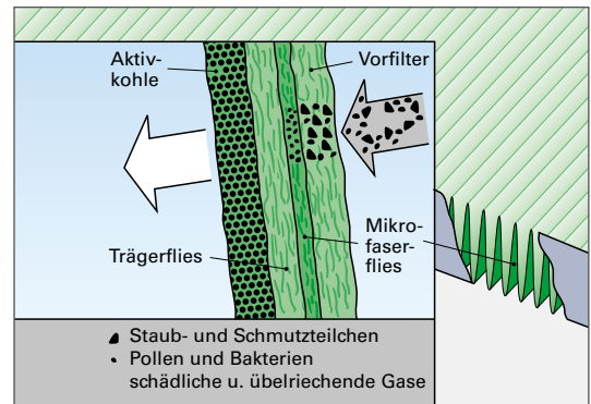
Bild 2: Aufbau eines Innenraumfilters
