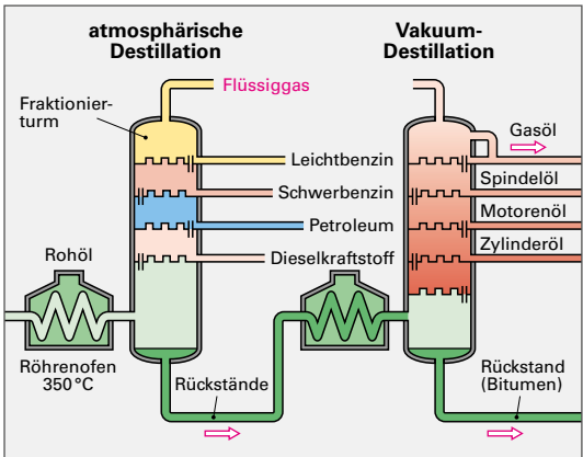
Bild 1: Destillieren von Rohöl
