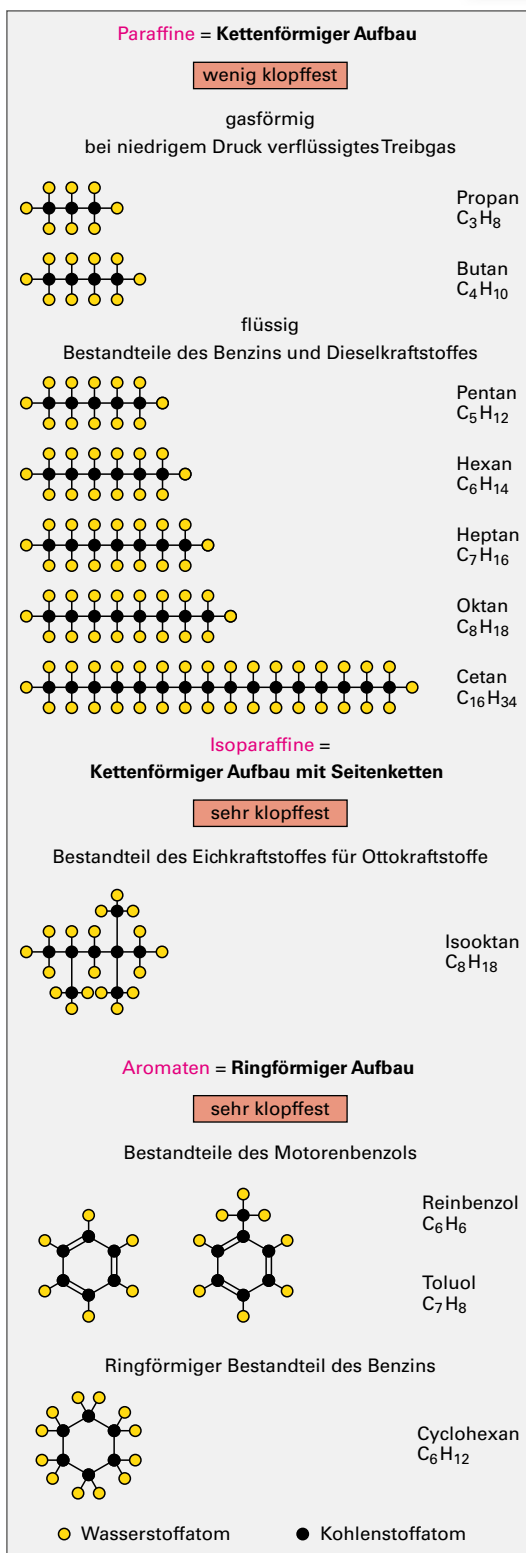
Bild 1: Aufbau der Kohlenwasserstoffmoleküle
