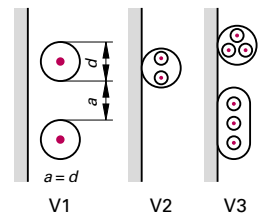
Verlegeanordnungen V
