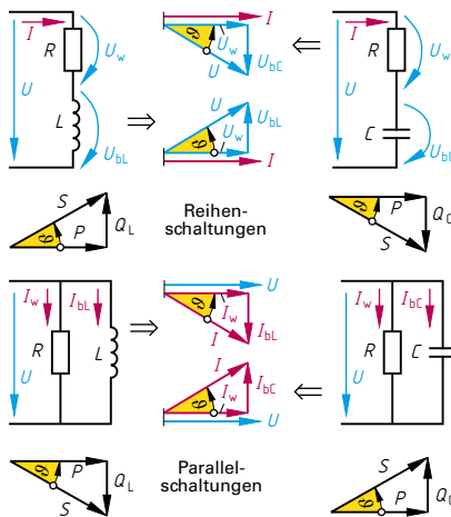
Schaltungen und Zeigerbilder
