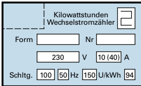
Leistungsschild eines Zählers
