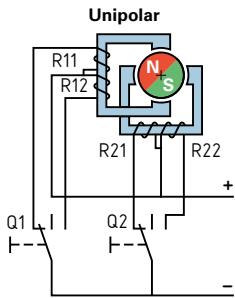
Zweistrang-Schrittmotoren
