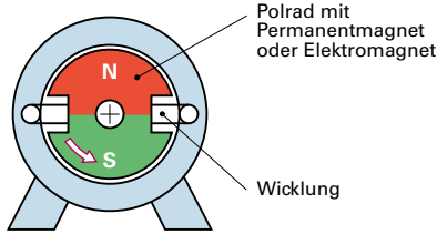
Innenpolmaschine mit einem Polpaar
