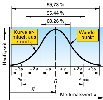
Normalverteilung
