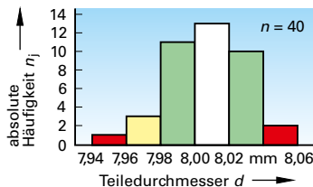
Histogrammdarstellung
