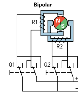
Die Schalter Q1 und Q2 sind z.B. Leistungstransistoren.
