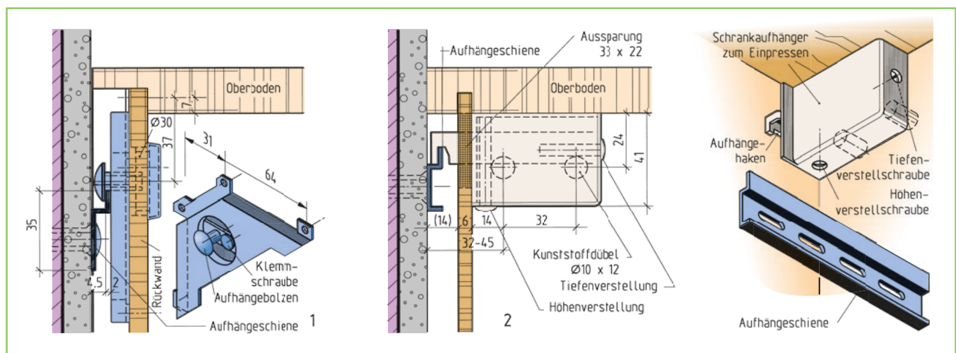
Bild 2: Aufhängemöglichkeit von Wandschränken wie Küchen-Oberschränken mit Beschlägen. 1 Hängebeschlag wird in die oberen Ecken des Möbels von hinten gegen die Korpuskanten geschraubt. Durch eine Bohrung in der Rückwand kann der Aufhängebolzen, der in eine Metallschiene fasst, verstellt und arretiert und der Schrank dadurch ausgerichtet werden. 2 Hängebeschlag wird oben in die hinteren Schrankecken gegen die Seiten gedübelt. Der höhen- und tiefenverstellbare Aufhängehaken fasst durch eine Aussparung der Rückwand in eine Metallschiene.
