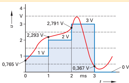
Bild 2: Abtasten eines analogen Signals
