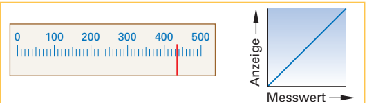
Bild 2: Analoge Darstellung eines Zeigerinstruments
