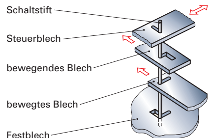
Bild 4: Mechanisches Speicherelement der Z1
