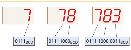
Bild 2: BCD-Zifferncodierung der Dezimalzahl 783
