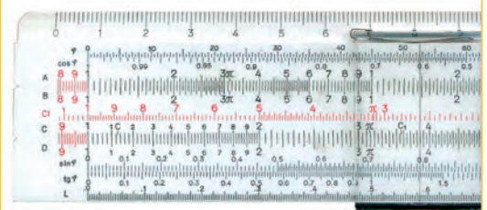
Bild 3: Rechenstab
