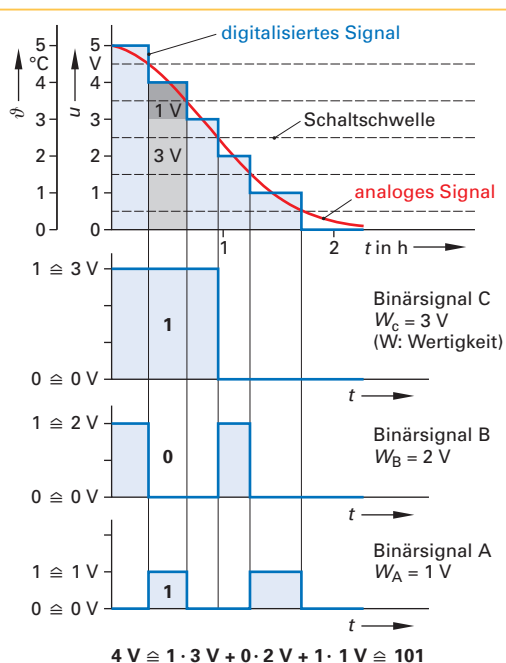
Bild 1: Digitalisiertes Temperatursignal
