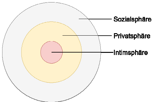
Abb. 17: Sphärentheorie
