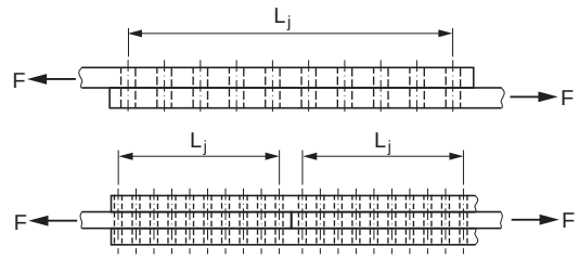
Bild 3.7. Lange Anschlüsse
