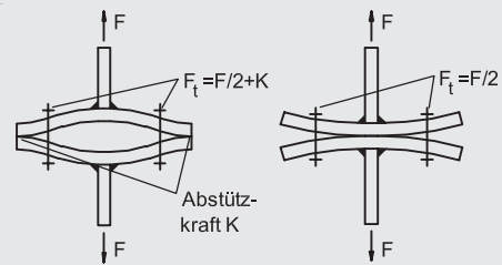
Beispiel für einen zugbeanspruchten T-Stoß
