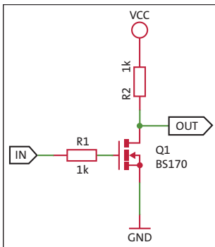
Abbildung 3.22 n-Kanal-FET als Schalter
