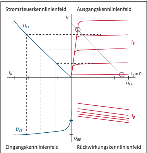
Abbildung 3.15 Transistor-Kennlinienfeld
