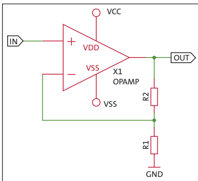
Abbildung 3.25 Nichtinvertierender Operationsverstärker
