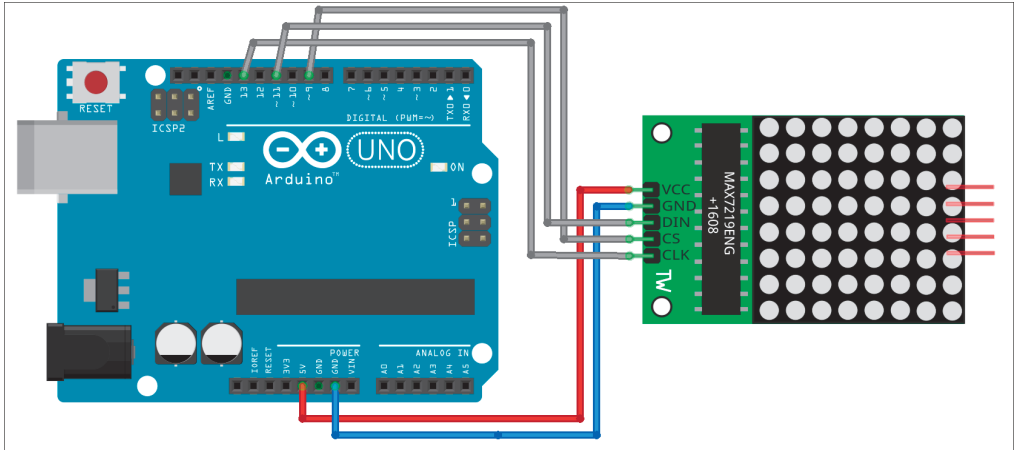
Abbildung 7.10 Dot-Matrix-Anzeige am Arduino Uno
