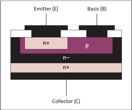
Abbildung 3.14 Aufbau des npn-Transistors
