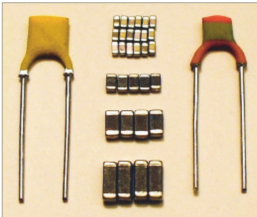
Abbildung 3.4 Keramik-Kondensatoren (Quelle: Elcap [CC BY-SA 3.0 ( http://creativecommons.org/licenses/by-sa/3.0/ )])
