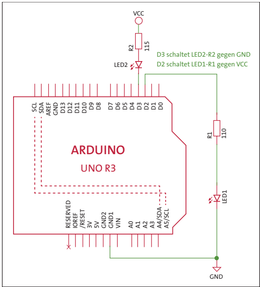
Abbildung 7.1 LEDs am Arduino Uno
