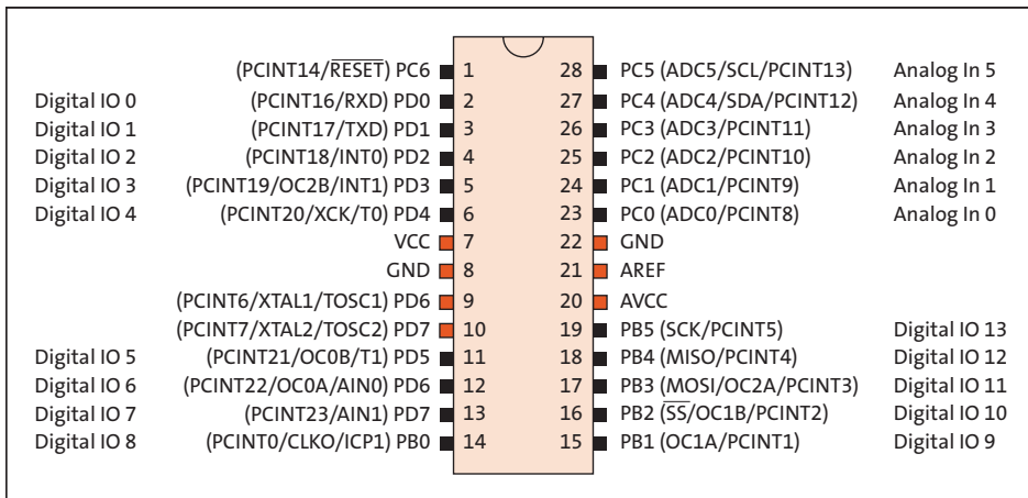
Abbildung 1.9 Anschlussbezeichnungen beim Arduino und ATmega328P
