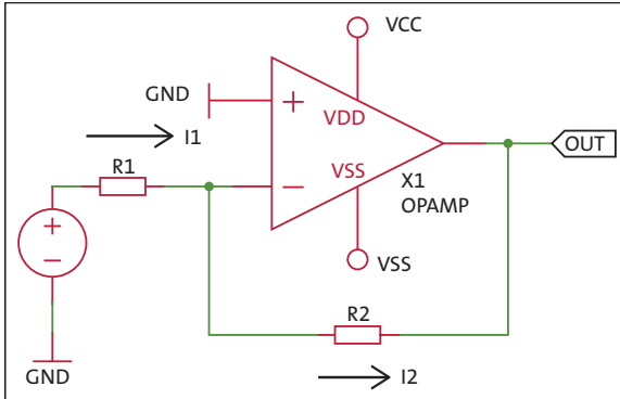
Abbildung 3.27 Invertierender Verstärker
