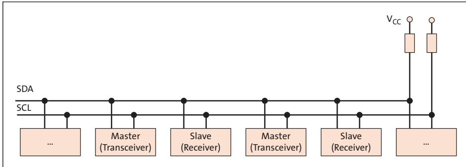
Abbildung 1.12 I 2 C-Bus-Netzwerk
