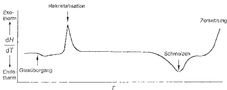
Abb. 1.3 Thermogramm eines teilkristallinen Polymers vom Glasübergang bis zur Zersetzung. [Aus: B. Tiede, Makromolekulare Chemie , Abb. 3, S. 13.]
