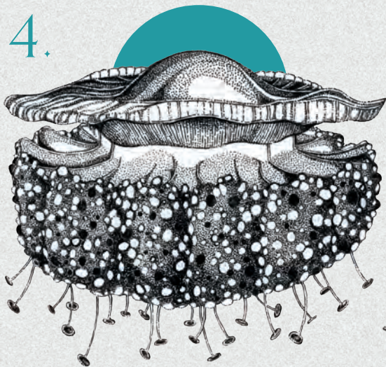
Spiegelei-Qualle
