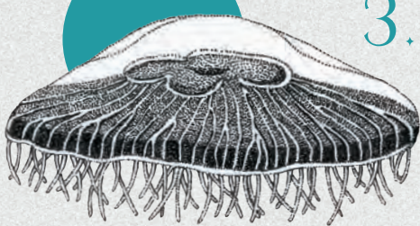
Ohrenqualle
