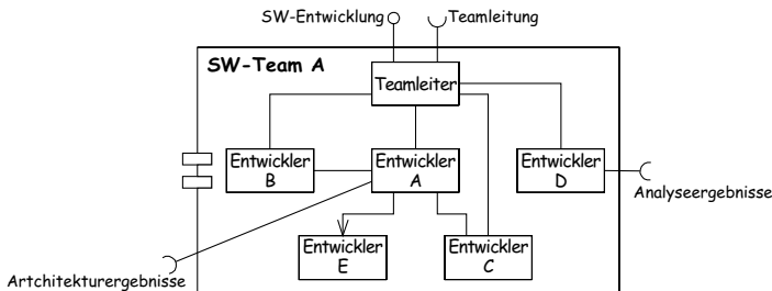
Abbildung 1.3: Zusätzlich zur Struktur aus Abbildung 1.2 finden wir innerhalb unserer Teilteams eine Mikrokommunikationsstruktur vor. (Beispielhafte Darstellung in UML: Alle Interfaces sind bidirektional.)
