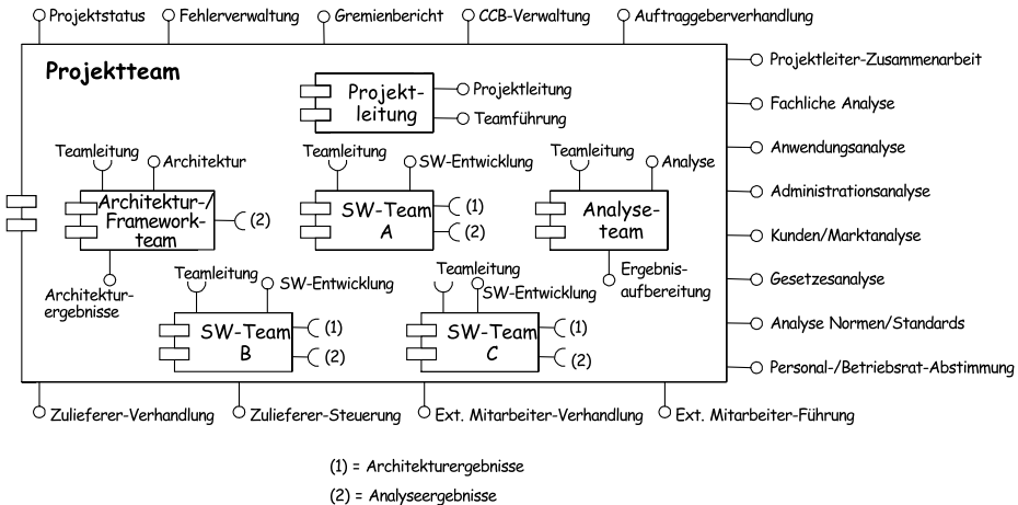
Abbildung 1.2: Die Verfeinerung der Projektstruktur aus Abbildung 1.1 führt zu einem komplexen Kommunikationsnetzwerk. (Beispielhafte Darstellung in UML: Alle Interfaces sind bidirektional.)
