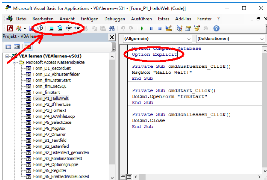
Abbildung 5.14: VBA-Code für das Ereignis Click auf dem Objekt cmdAusfuehren des Formulars P1-HalloWelt.
