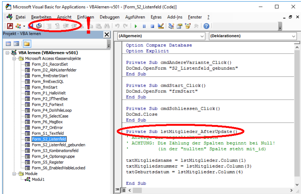
Abbildung 5.12: VBA-Code für das Ereignis AfterUpdate auf dem Objekt lstMitglieder des Formulars Form_S2_Listenfeld .
