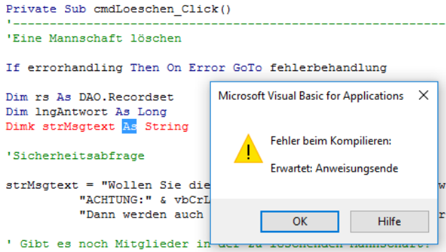
Abbildung 5.4: Das VBA-Schlüsselwort Dim wurde falsch geschrieben.
