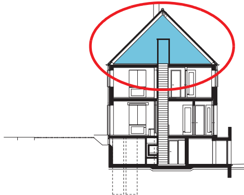
Schnitt
