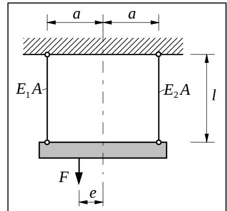
Bild 1.2: Starrer Balken, aufgehängt an zwei Stäben aus unterschiedlichem Material
