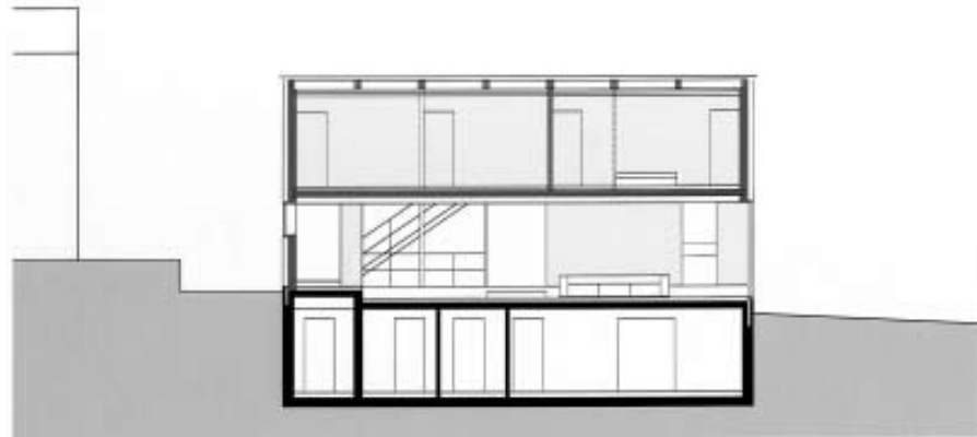
Schnitt 2
