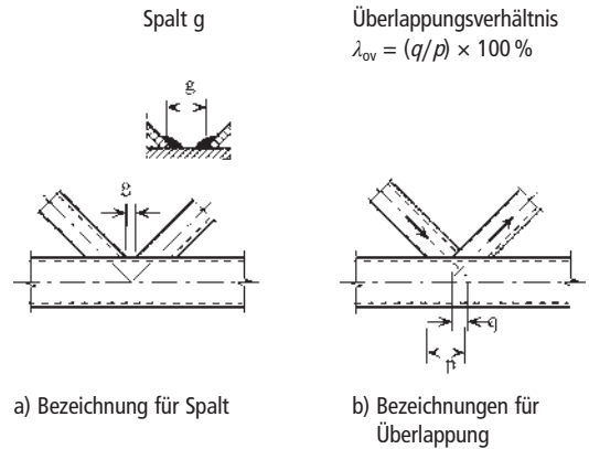
Bild 1.3. Knotenanschlüsse mit Spalt und mit Überlappung
