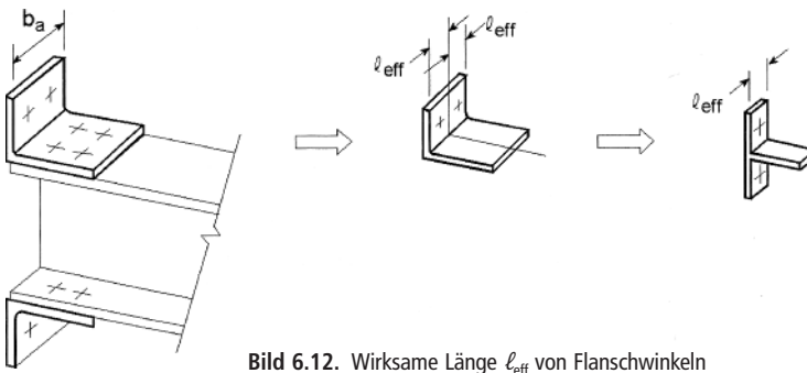
Bild 6.12. Wirksame Länge l_{\text{eff}} von Flanschwindeln
