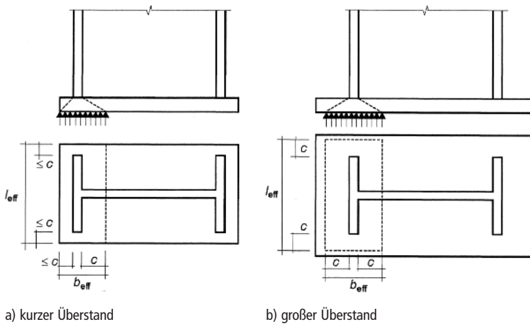
Bild 6.4. Fläche des äquivalenten T-Stummels mit Druckbeanspruchung
