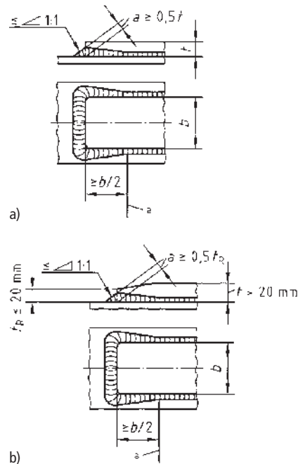
Bild NA.4. Vorbinden zusätzlicher Gurtplatten
