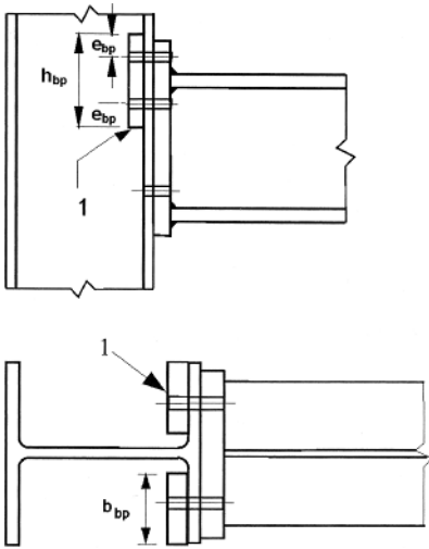
Legende h_{bp} \geq \sum \ell_{eff,1} 1 Verstärkungsblech e_{bp} \geq 2d
