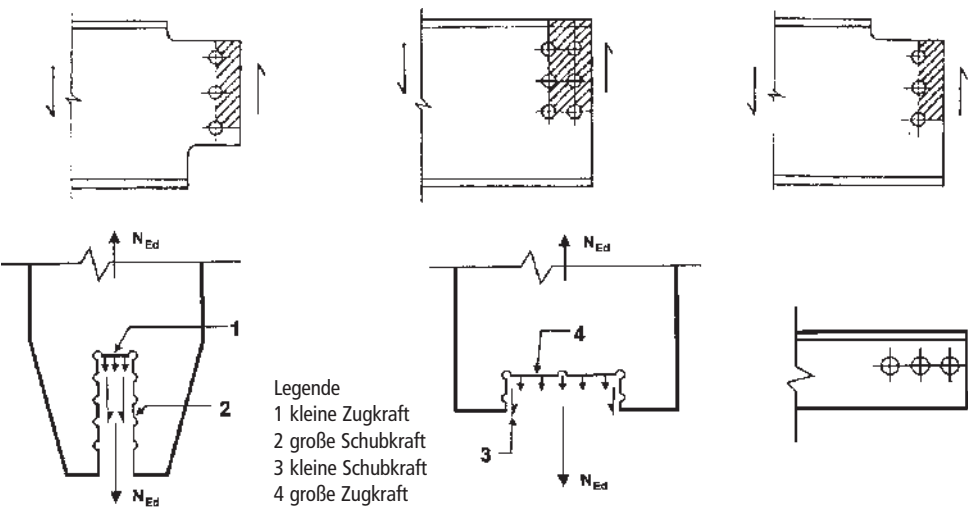
Bild 3.8. Blockversagen von Schraubengruppen
