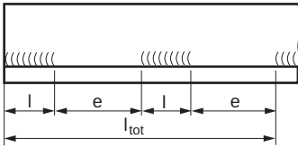
Bild 4.7. Berechnung der Scherkkräfte auf unterbrochen geschweißte Schweißnähte
