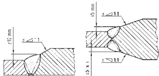
a) Einseitig bündiger Stoß
