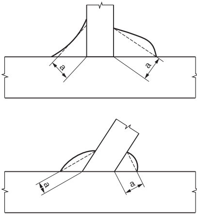
Bild 4.3. Kehl-nahtdicke
