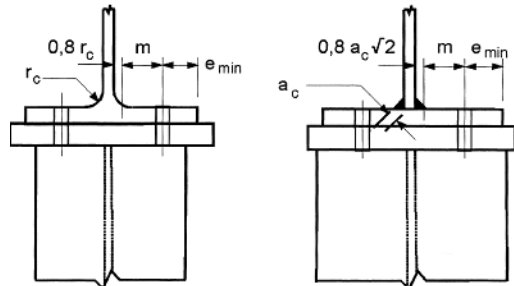
b) Geschweißtes Stirnblech breiter als der Stützenflansch
