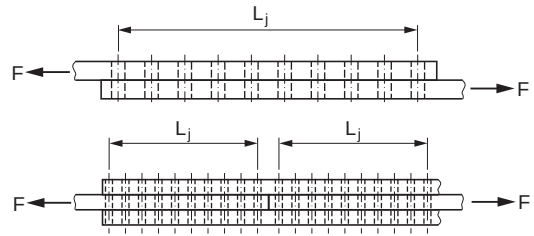
Bild 3.7. Lange Anschlüsse
