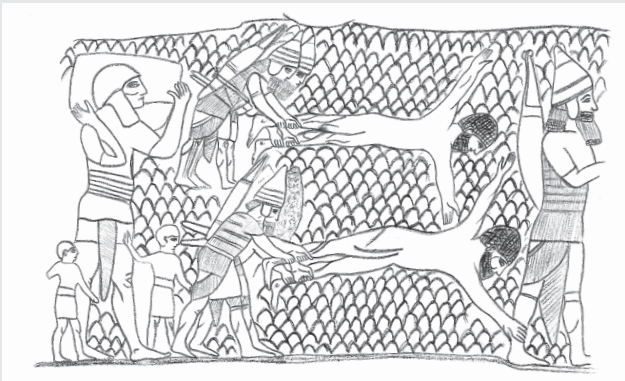
Abb. 2: Häutung
