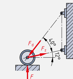
Kräfteplan
