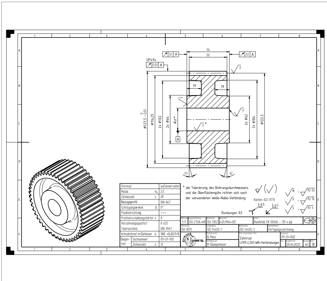
Bild 1: Zahnrad
