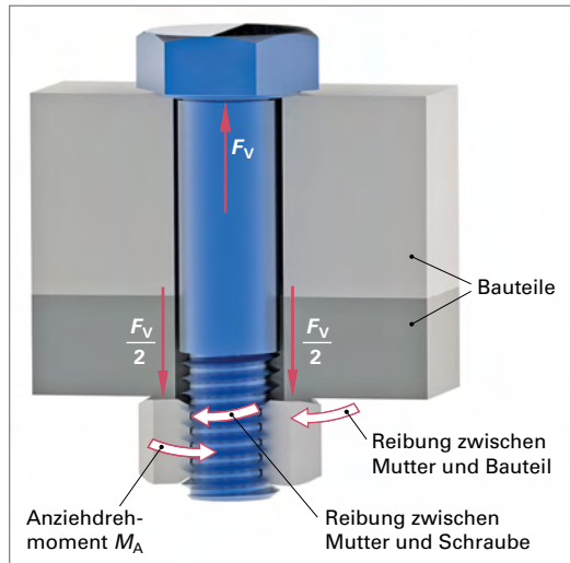
Bild 1: Reibung am Gewinde
