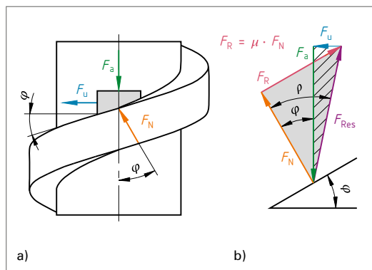
Bild 3: Kräfte an den Gewindeflanken mit Reibung (Mutter bewegt sich nach unten)
