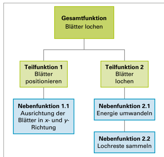
Bild 2: Teil- und Nebenfunktionen des Bürolochers
