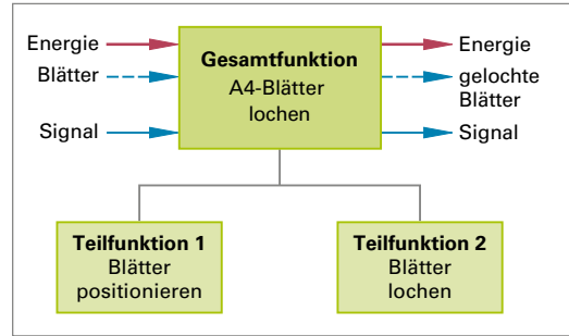
Bild 1: Gesamt- und Teilfunktionen am Beispiel eines Bürolochers
