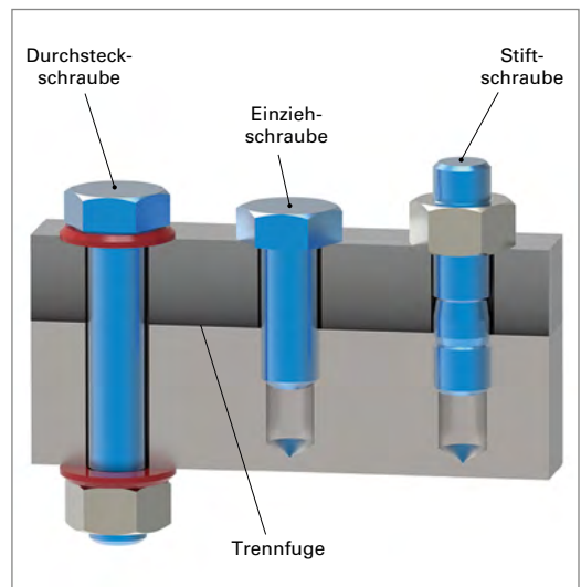
Bild 2: Befestigungsarten von Schraubenverbindungen
