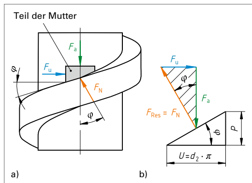
Bild 2: Kräfte an den Gewindeflanken ohne Reibung (Mutter bewegt sich nach oben)
