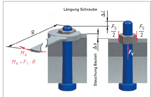
Bild 1: Anziehen der Schraubenverbindung
