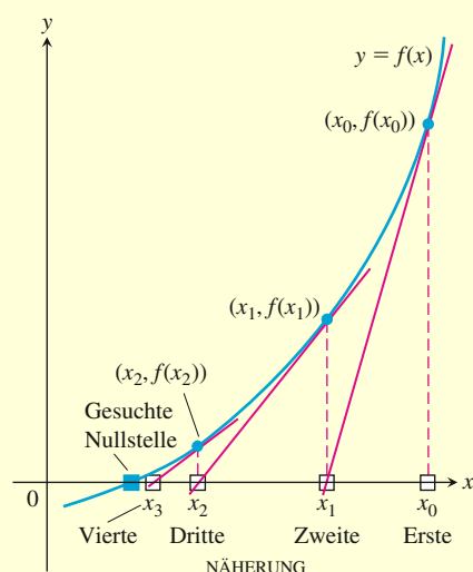
Abbildung 4.41 Das Newton-Verfahren beginnt mit einem geratenen Startwert x_0 und verbessert (im Idealfall) die Näherung in jedem Schritt.
